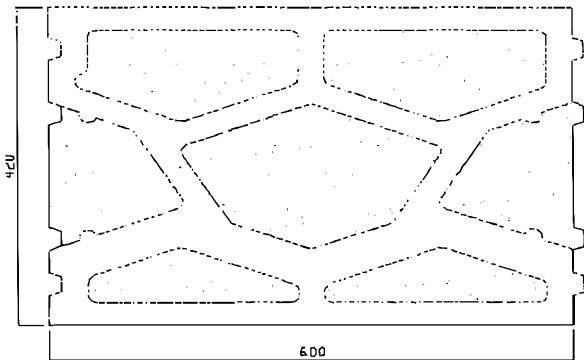
GT H - ROVNÝ
